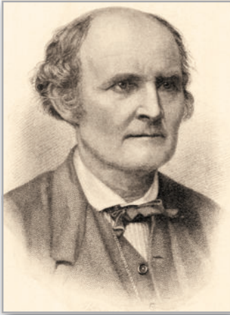
Arthur Cayley (1821–1895)
